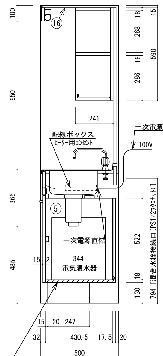
電気温水器用底板補強
