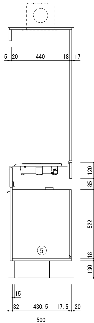
電気温水器用底板補強
