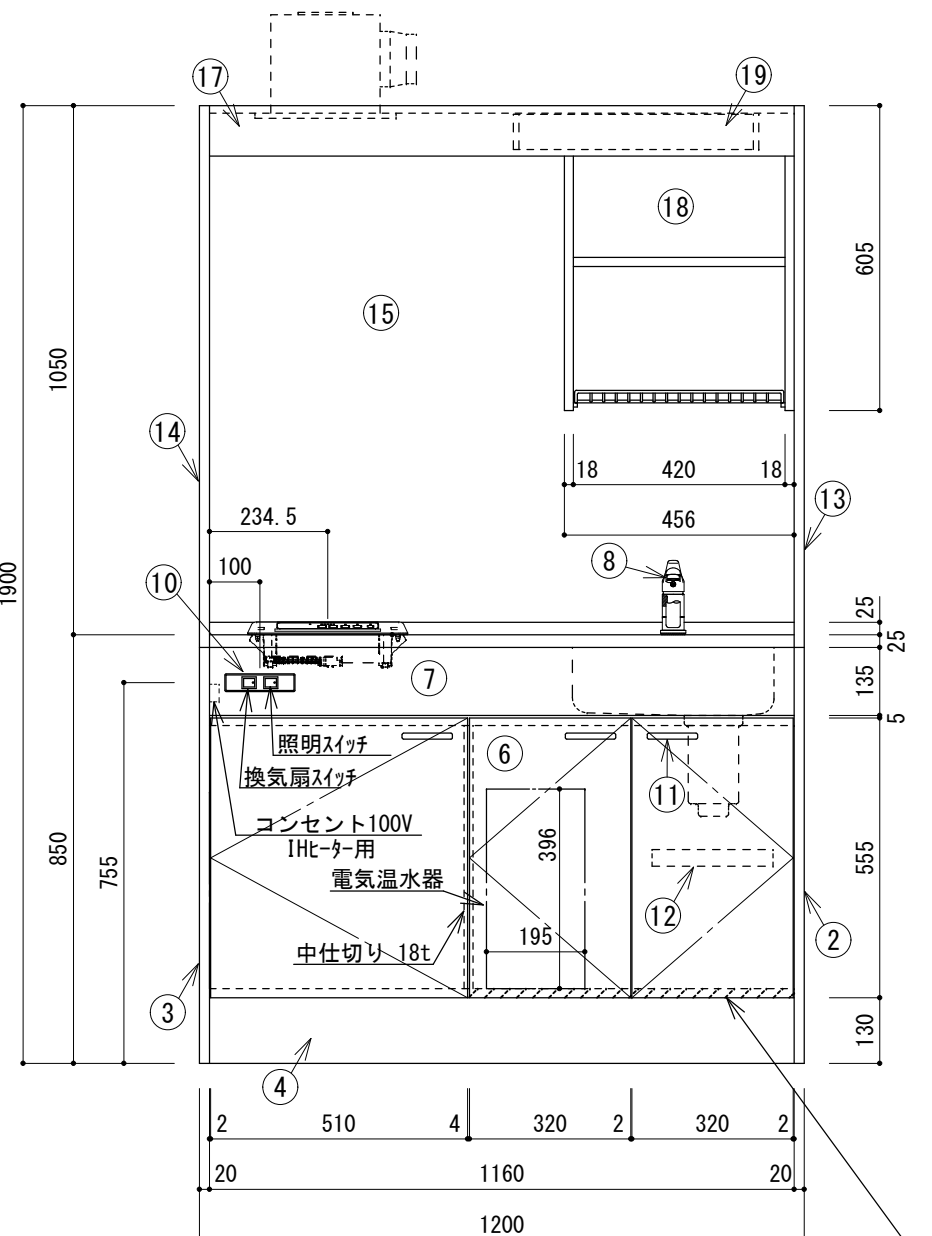
電気温水器用底板補強
