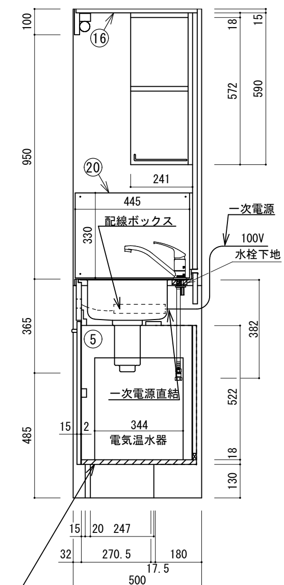
電気温水器用底板補強
