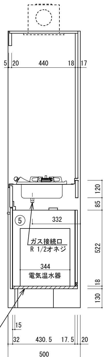
電気温水器用底板補強
