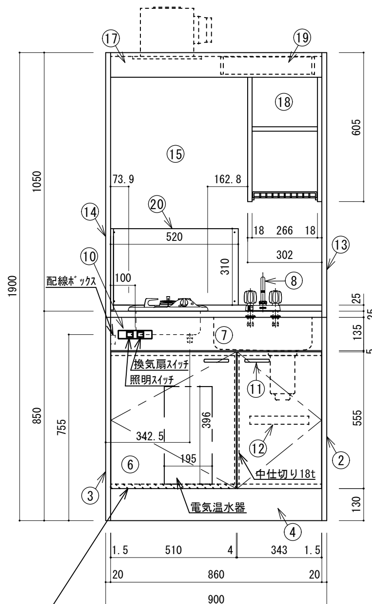
電気温水器用底板補強
